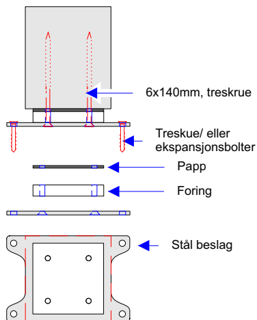
EKS-Søylefot-beslag
